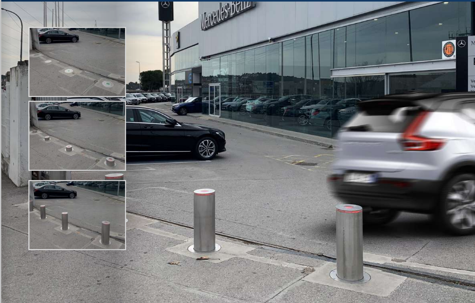
Instalación de una PILONA AUTOMÁTICA de 600mm de altura, con doble semáforo; en la salida sobre un poste y en el conjunto de totem con semáforo integrado, interfono y lector de tarjetas.
